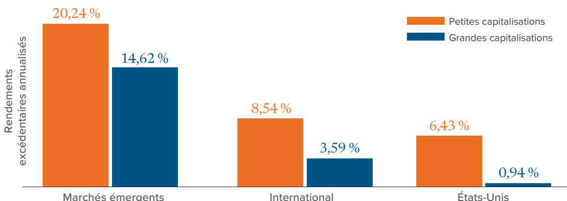
FIGURE 2 – Efficacité quantitative de l’alpha, septembre 2003 – décembre 2024
